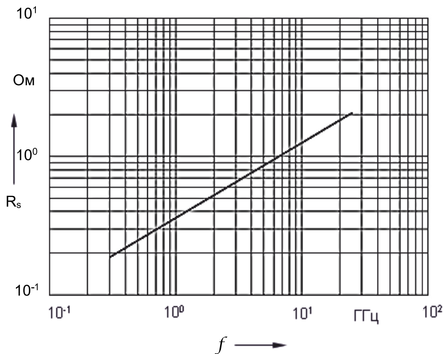
Рис.3 – Зависимость эквивалентного последовательного сопротивления R_s конденсаторов от частоты
