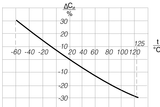
Характер зависимости емкости фильтров группы M3300 от температуры
