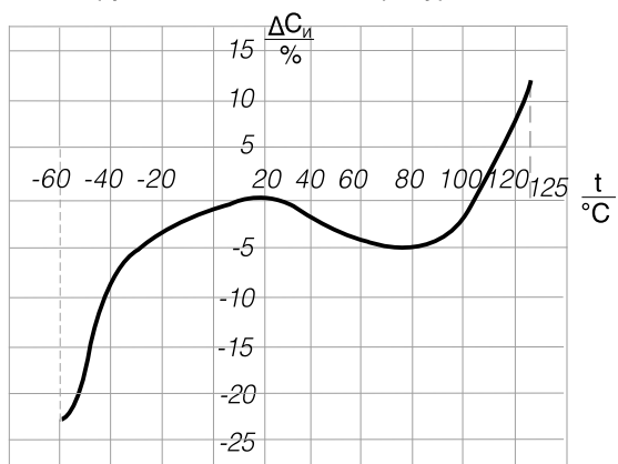
Характер зависимости емкости фильтров группы H30 от температуры
