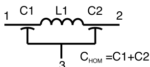
Электрическая схема фильтров Б24
