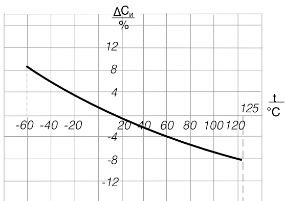
Характер зависимости емкости фильтров группы M750 от температуры
