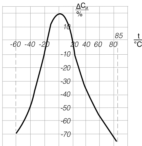
Характер зависимости емкости фильтров группы H90 от температуры
