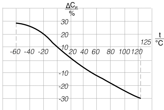
Характер зависимости емкости фильтров группы M2200 от температуры
