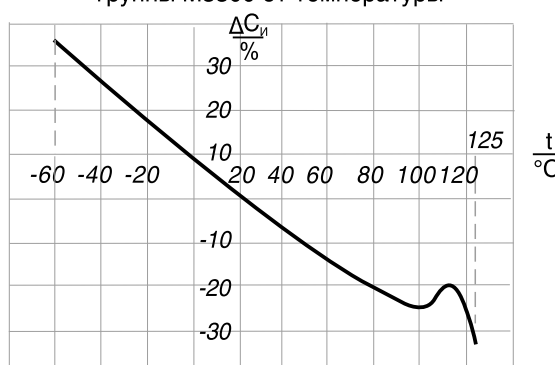
Характер зависимости емкости фильтров группы H50 от температуры
