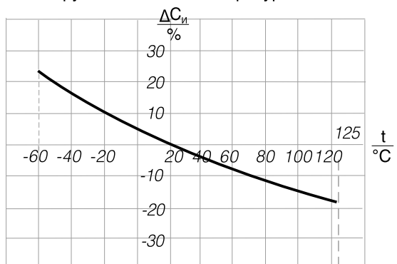
Характер зависимости емкости фильтров группы M1500 от температуры
