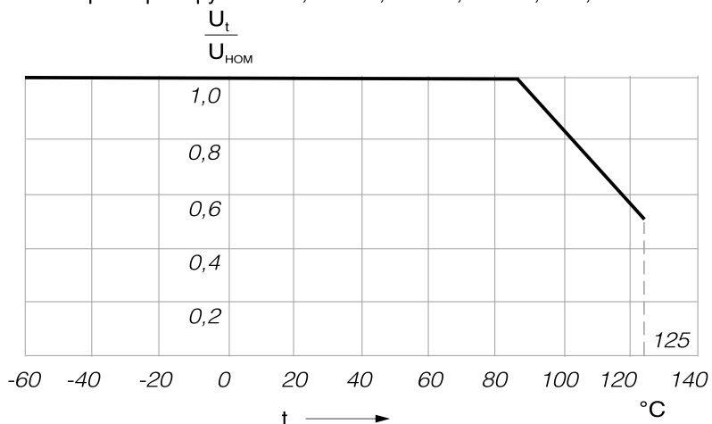
Зависимость допускаемого напряжения от температуры фильтров групп М750, М1500, М2200, М3300, Н30, Н50
