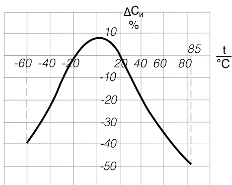
Характер зависимости емкости фильтров группы H70 от температуры
