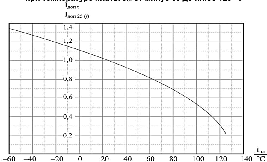
Рис.3 – Зависимость допускаемого реактивного тока I_{\text{доп } t} (эффективное значение) при температуре платы t_{\text{пл}} от минус 60 до плюс 125 °C
