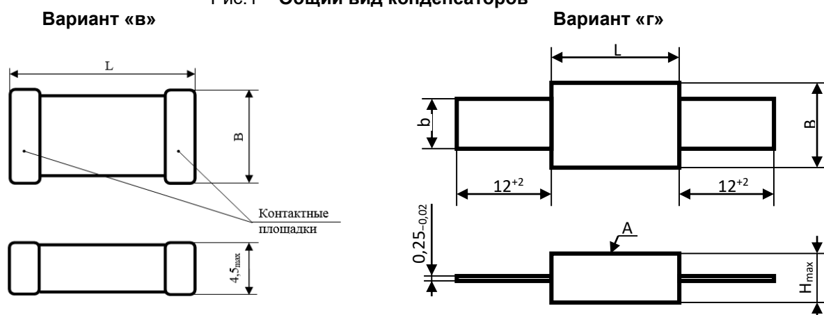
Рис.1 – Общий вид конденсаторов
