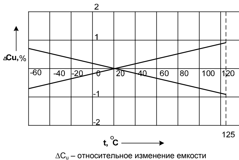
Характер зависимости емкости конденсаторов от температуры
