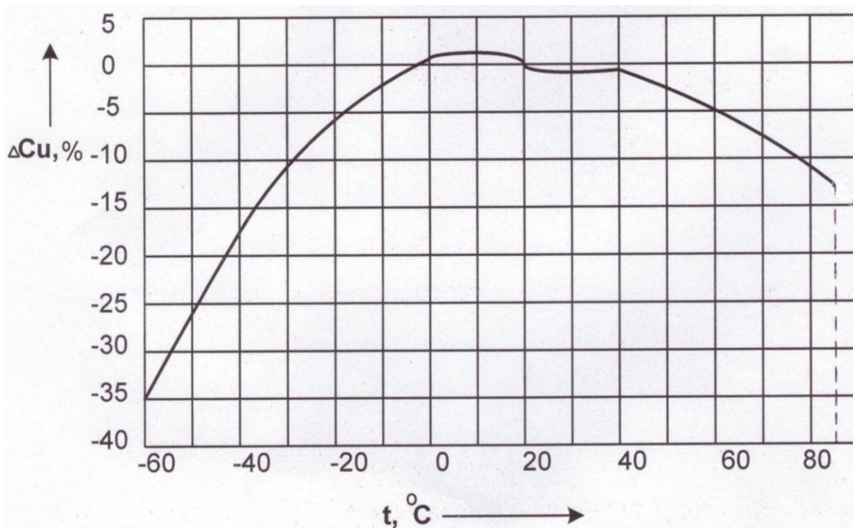
Характер зависимости емкости конденсаторов группы Н50 от температуры
