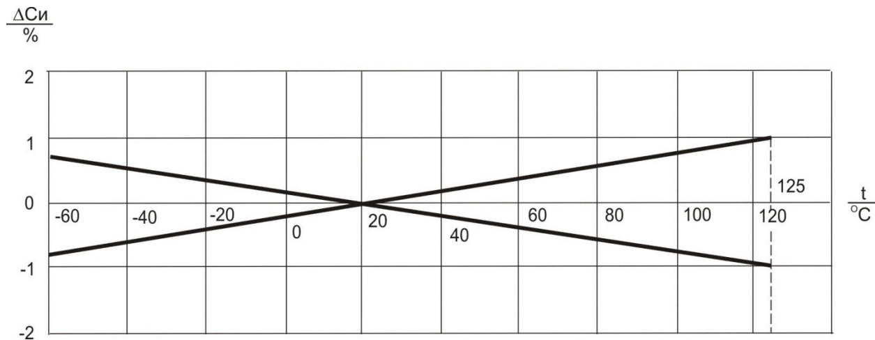
Характер зависимости емкости конденсаторов группы МПО от температуры
