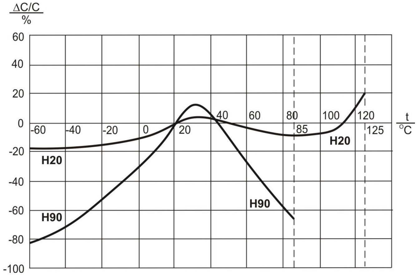
Рис.3 - Характер зависимости изменения емкости конденсаторов от температуры
