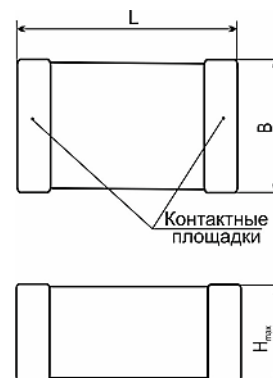
Рис.1 - Общий вид конденсатора
