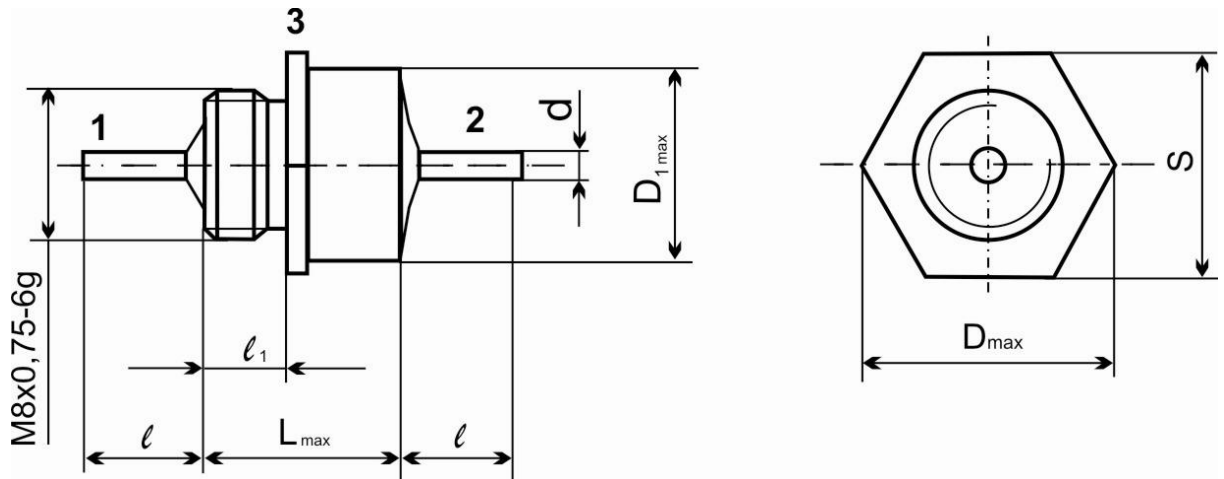
Рис. 1 С-фильтры Б26 – 1 (15 А и 25 А), LC-фильтры Б26-2 (15 А), Рі-фильтры Б26-3 (15 А и 25 А)
