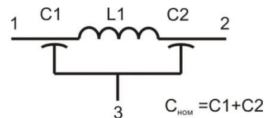
Вариант 3 Б26-3 с I_{НОМ} = 15; 25 \text{ А}
